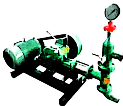
BW60-8砂浆注浆泵
