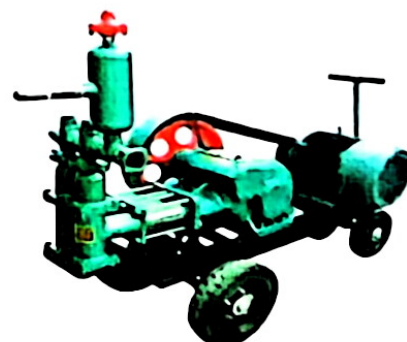
BW70-10砂浆注浆泵
