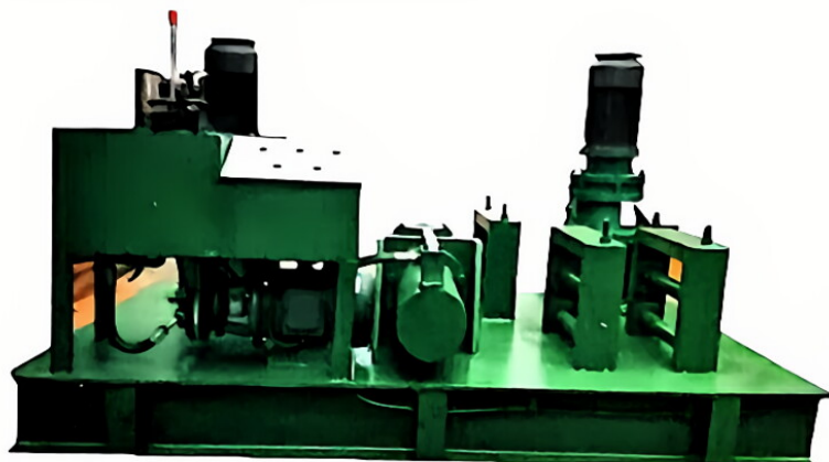
WGJ-250弯拱机
