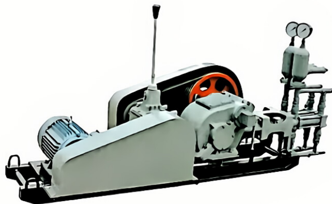
矿用双液变量注浆泵
