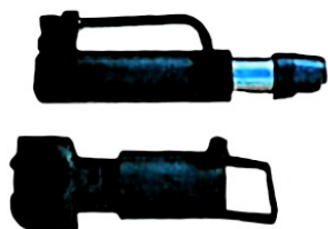
退锚器头、千斤顶
