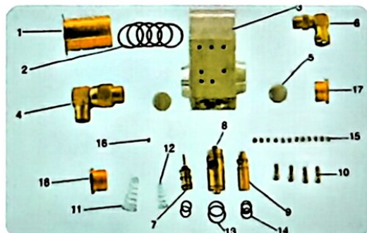
阀块分解图
