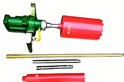
气动手持式水钻
